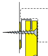
Det S4: Kiinnitys polyuretaani- liimamassalla tai ruuvilla
